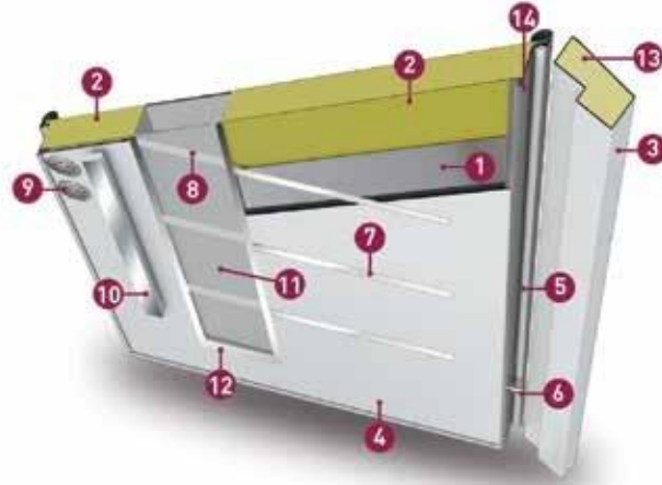
Kesit Görünüş / Section view
