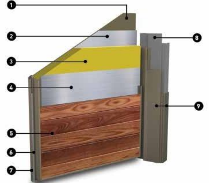
Kesit Görünüş | Section View
