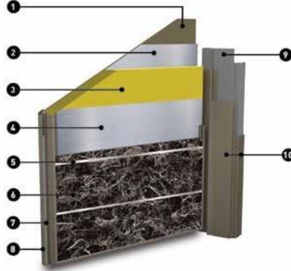
Kesit Görünüş | Section View
