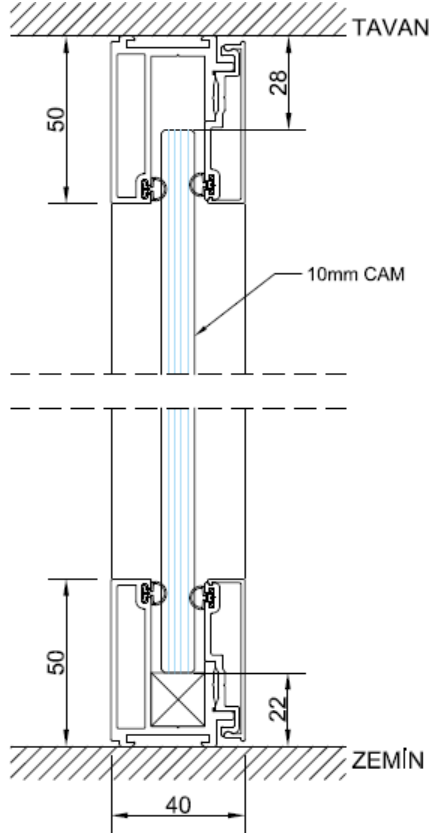
SİSTEM KESİTİ
